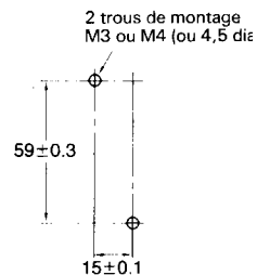
Trous de montage
