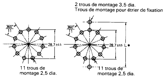
Dimensions des trous de montage pour modèle MK
